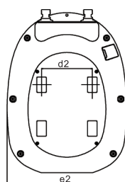
Вид сзади
