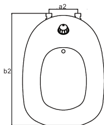
Вид спереди
